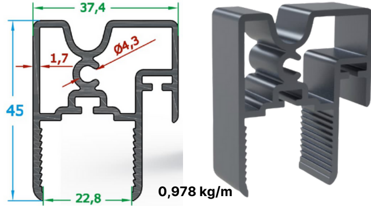
Tırnaklı Kanat Profili/Latch Wing Profile
