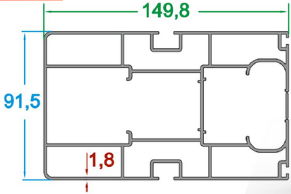
90'lık Orta Ray Profili/90 Medium Rail Profile
