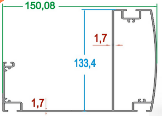
Ince Oluk Profili (Ustten Tek Kanallı)/Thin Gutter Profile
