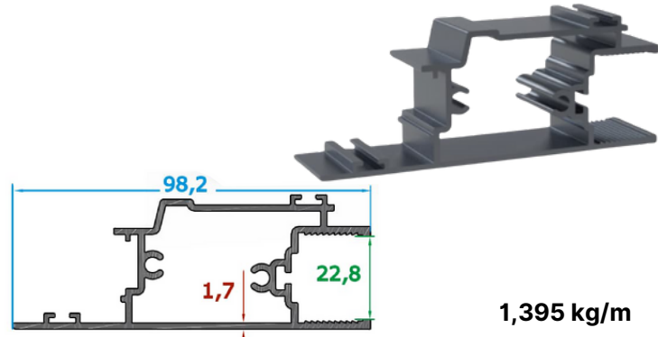
Alt Kanat Dikme Profili/Bottom Wing Strut Profile
