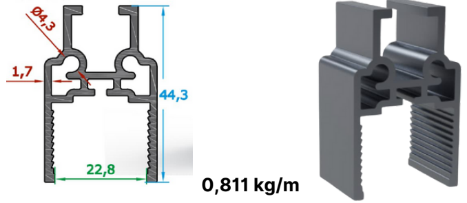
Kanat Dikey Profili/Wing Vertical Profile
