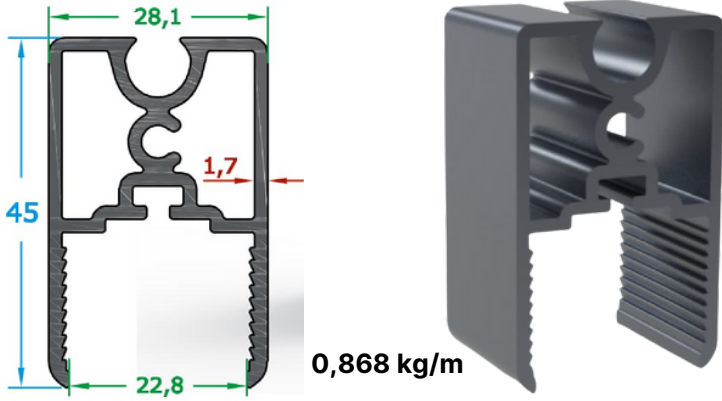
Tırnaksız Üst Baza Profili/Top Plinth Profile Without Nail
