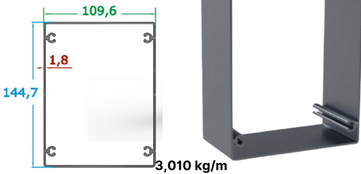
110x145 Dikme Profili/110x145 Strut Profile
