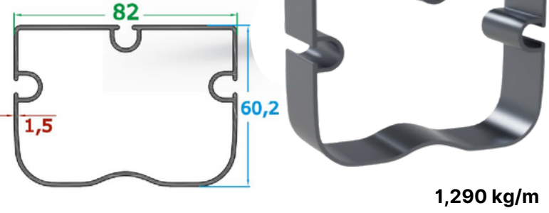
Damla Kalın Korniş Profili/Drop Thick Cornice Profile
