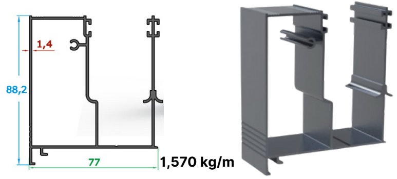
Üst Orta Yaprak Profili/Upper Middle Leaf Profile
