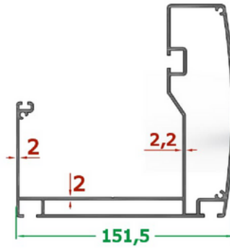
Kalın Oluk Profili (İçten Tek Kanallı)/Thick Gutter Profile
