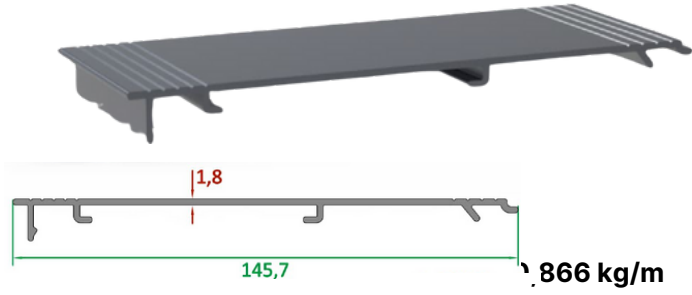
Motor Kutusu Kapağı Profili/Engine Box Cover Profile
