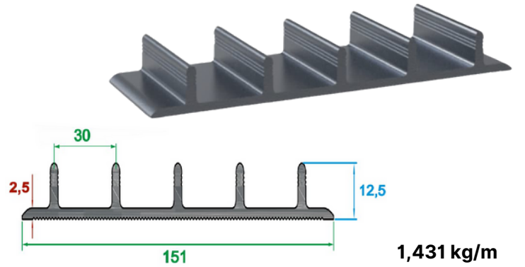
Eşiksiz 5'li Kasa Profili/5 Case Profile Without Threshold
