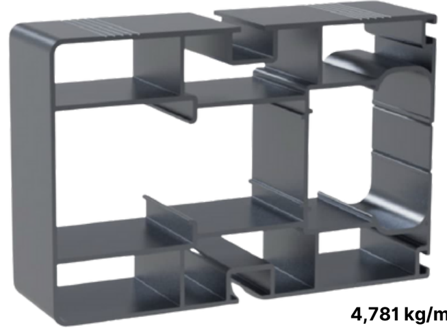
90'lık Orta Ray Profili/90 Medium Rail Profile
