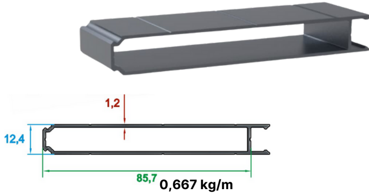
3'lü Yan Profili/3 Side Profile
